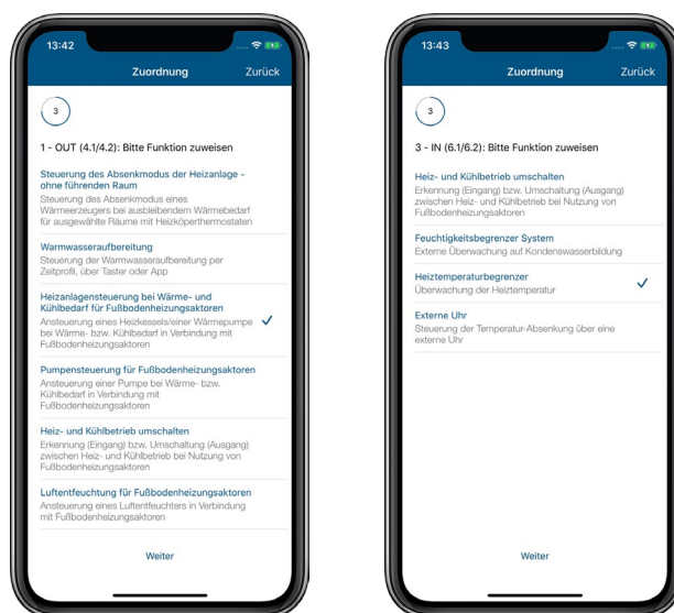
Abbildung 49: Screenshot Konfiguration HmIP-MIOB für Temperaturbegrenzung
